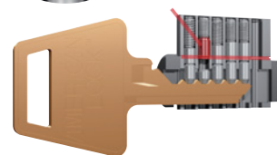
Pasador cónico inverso
